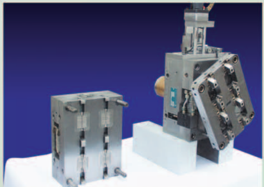
Spritzgießwerkzeug Schließklappen 2 Komponentenwerkzeug mit Indexplatte Formgröße: 396 x 296 x 390
